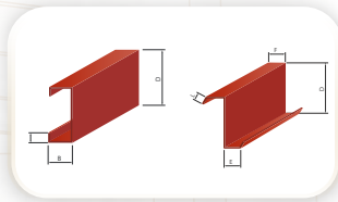
Xà gỗ C - Xà gỗ Z
