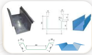
Máng xối inox - Máng xối tôn mạ màu
