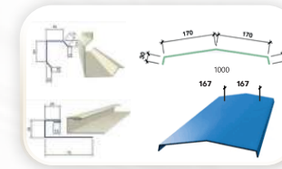
Diêm góc - Nẹp diêm - Úp nóc
