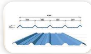
Tôn 05 sóng
