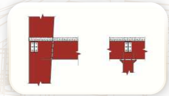
Hệ khung có sàn theo chi tiết cấu tạo
