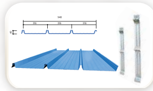
Tôn Klip-Lock - Đại Klock
