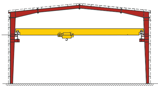
Cầu trục chạy trên ray
