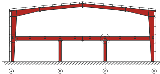
Hệ khung có sàn (mặt cắt)
