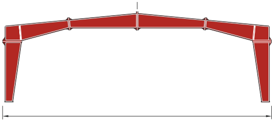
Hệ khung một nhịp không cột giữa
