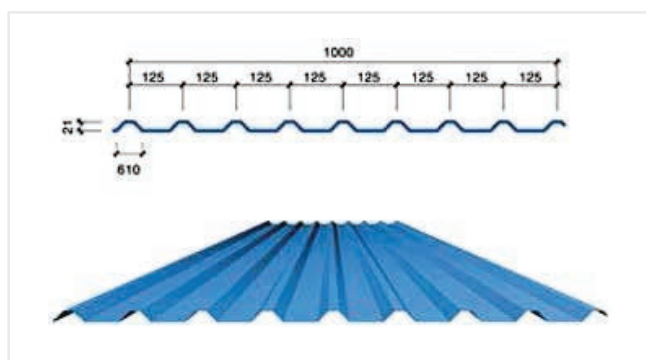
Tôn 09 sóng
