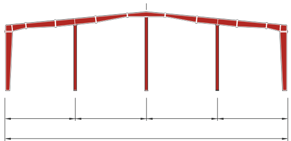
Hệ khung một nhịp nhiều cột giữa
