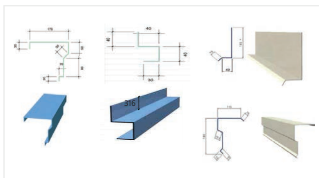
Diềm hồi - Diềm chắn nước - Diềm đầu hồi
