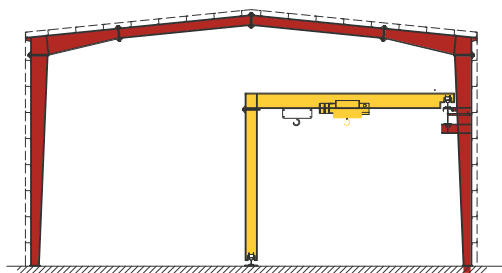
Cổng trục chung cột
