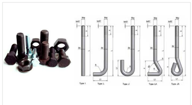
Bulon liên kết - Bulon Móng
