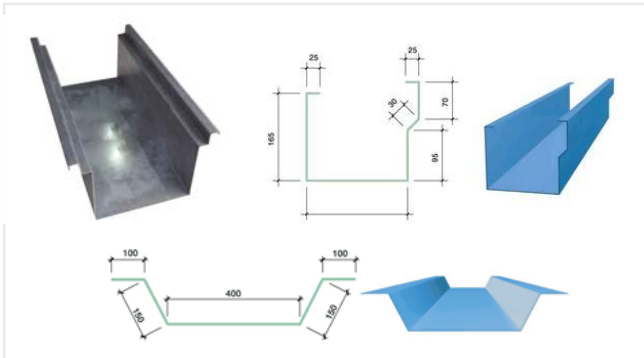
Máng xối inox - Máng xối tôn mạ màu
