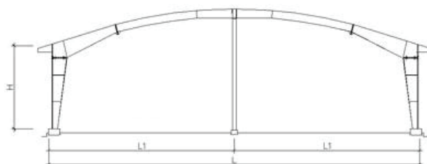
Khung kèo vòm 2 nhịp
