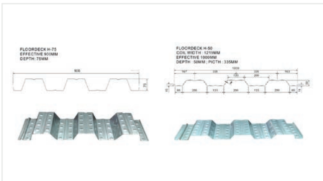
Sàn deck
