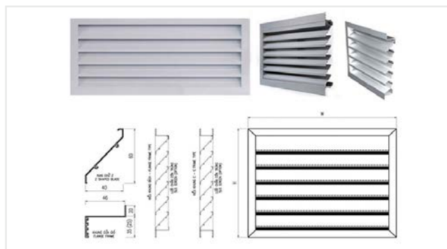
Lam gió
