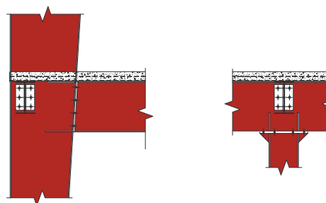
Hệ khung có sàn (chi tiết cấu tạo)
