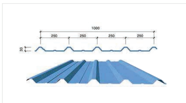
Tôn 05 sóng
