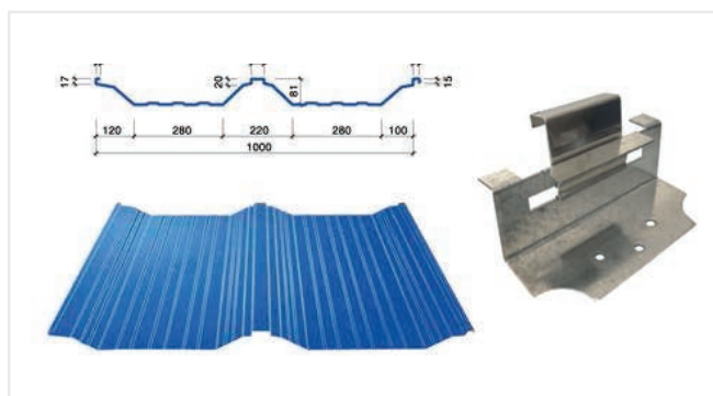
Tôn Lockseam - Đại seam
