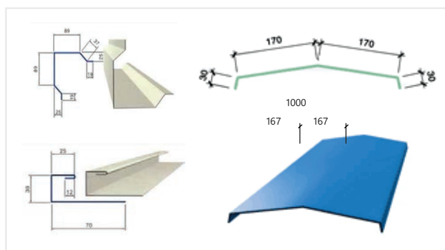
Diềm góc - Nẹp diềm ô cửa khung - Úp nóc
