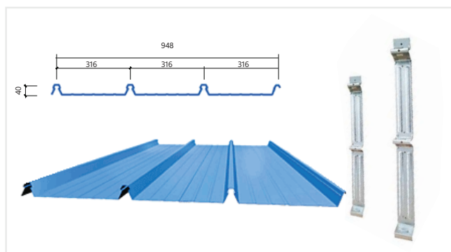
Tôn Klip-Lock - Đại lock
