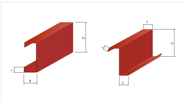
Xà gồ C - Xà gồ Z
